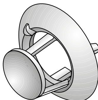
TERMINAL SIMPLE DE ASPIRACIÓN Y DESCARGA PARA TUBOS SEPARADOS \varnothing 35 MM
