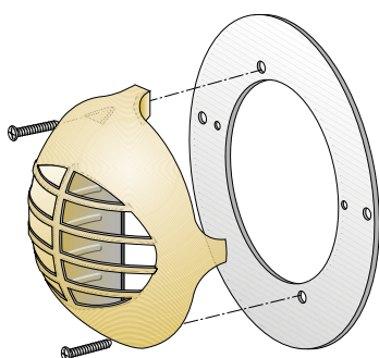
TERMINAL Y BRIDA DE ASPIRACIÓN Y DESCARGA ESTÁNDAR
